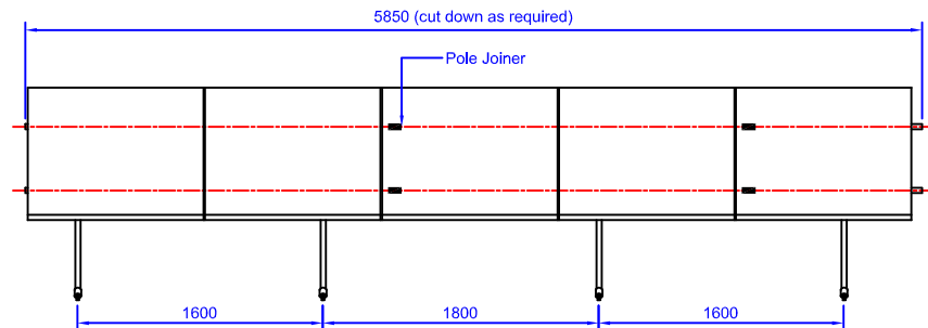
5 Module structure
