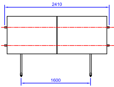
2 Module structure
