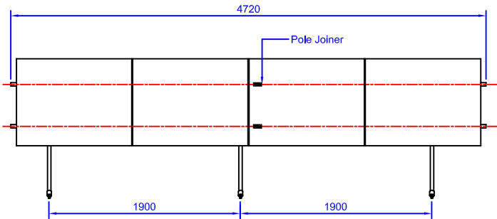
4 Module structure
