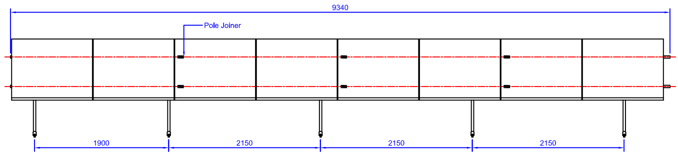
8 Module structure
