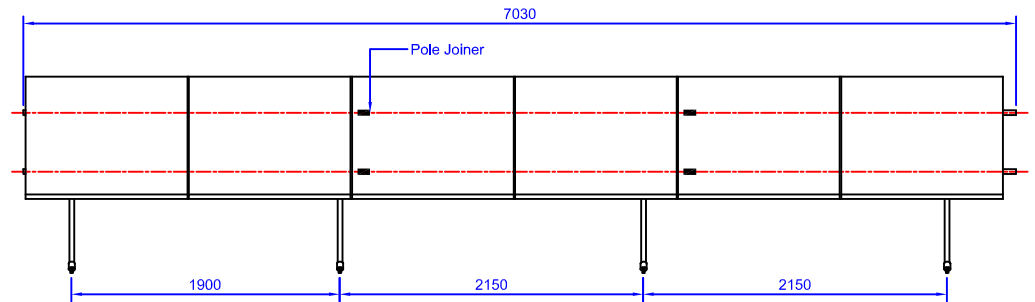
6 Module structure
