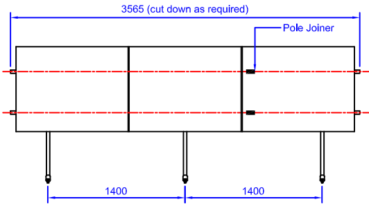
3 Module structure
